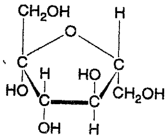
Fructose
